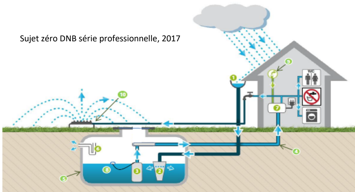
Figure 1 : Installation technique de récupération et de distribution d'eau de pluie.
